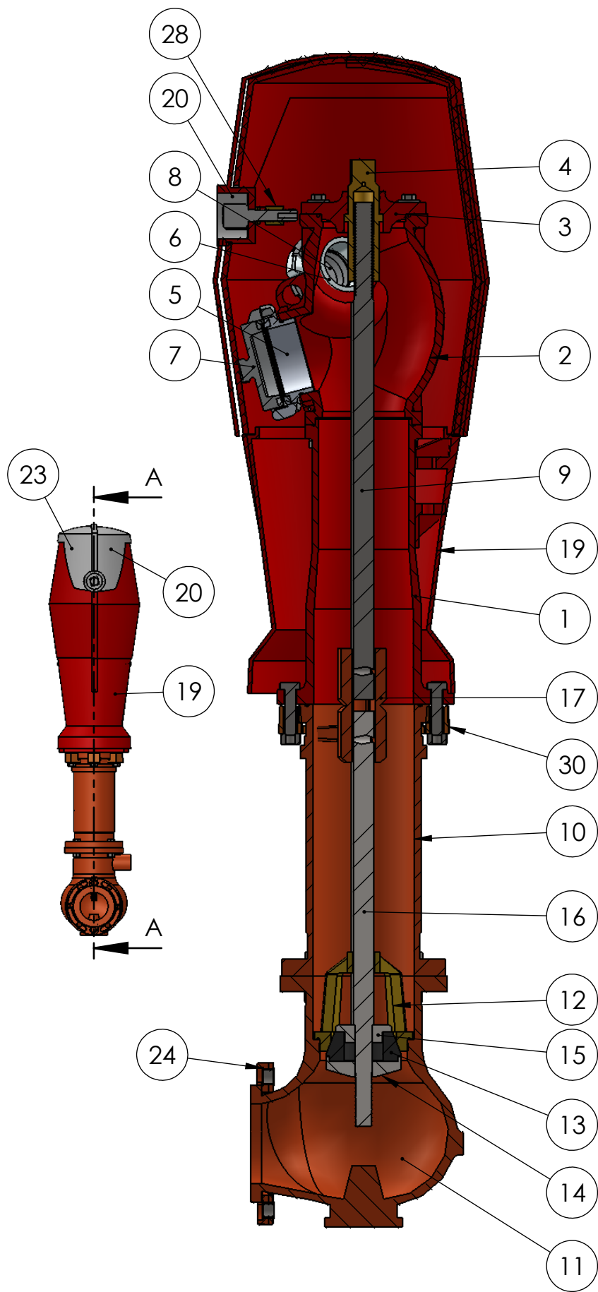
SECCIÓN A-A
