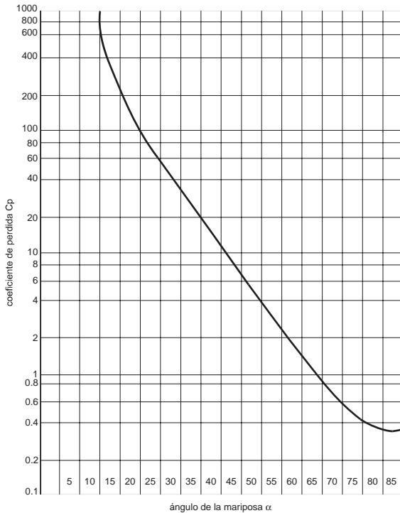
coeficiente de pérdida de Cp de válvula de mariposa CP Loss coefficient
