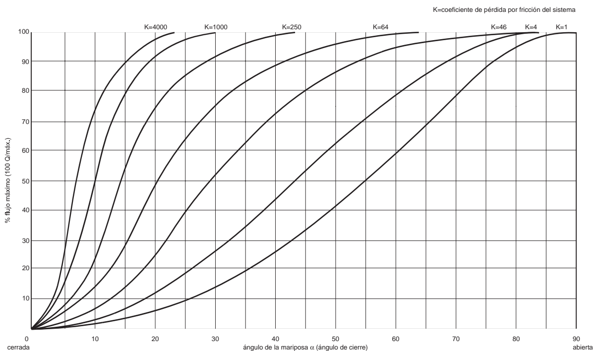
características de control de las válvulas de mariposa control features of butterfly valves
