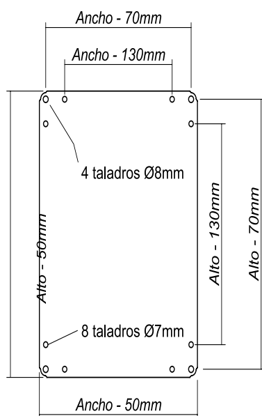
Vista de placa de montaje
