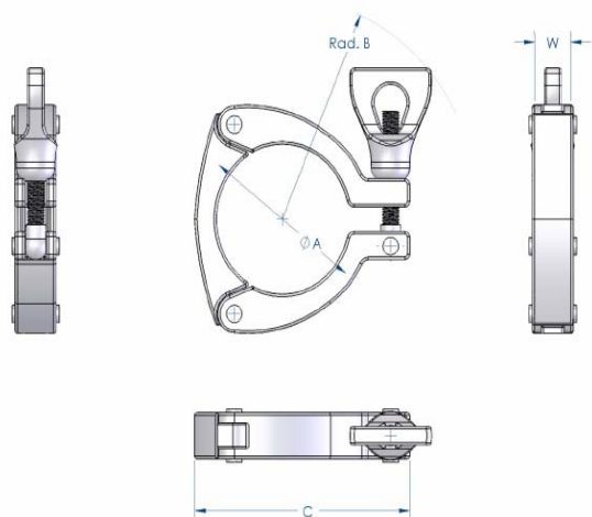
Abrazadera 3 Cuerpos
