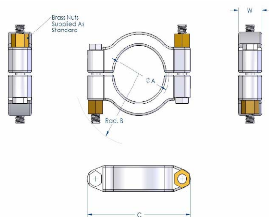
Abrazadera SSH
