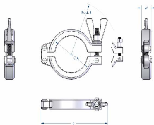
Abrazadera SH
