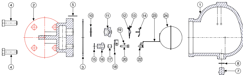
Mod. 243 1/2", 3/4" y 1"
