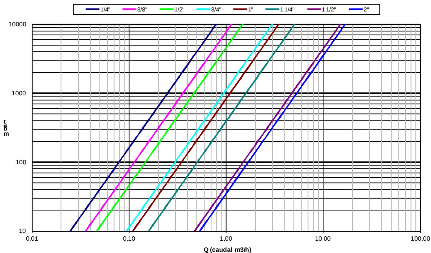
DIAGRAMA DE PERDIDA DE CARGA / HEADLOSS CHART VÁLVULAS DE AGUJA / NEEDLE VALVES
